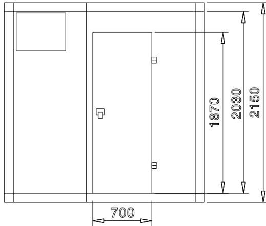
Zij aanzicht
